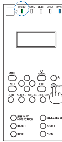
投影机上 SHUTTER 指示灯
